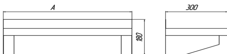
Вариант сборки 2
